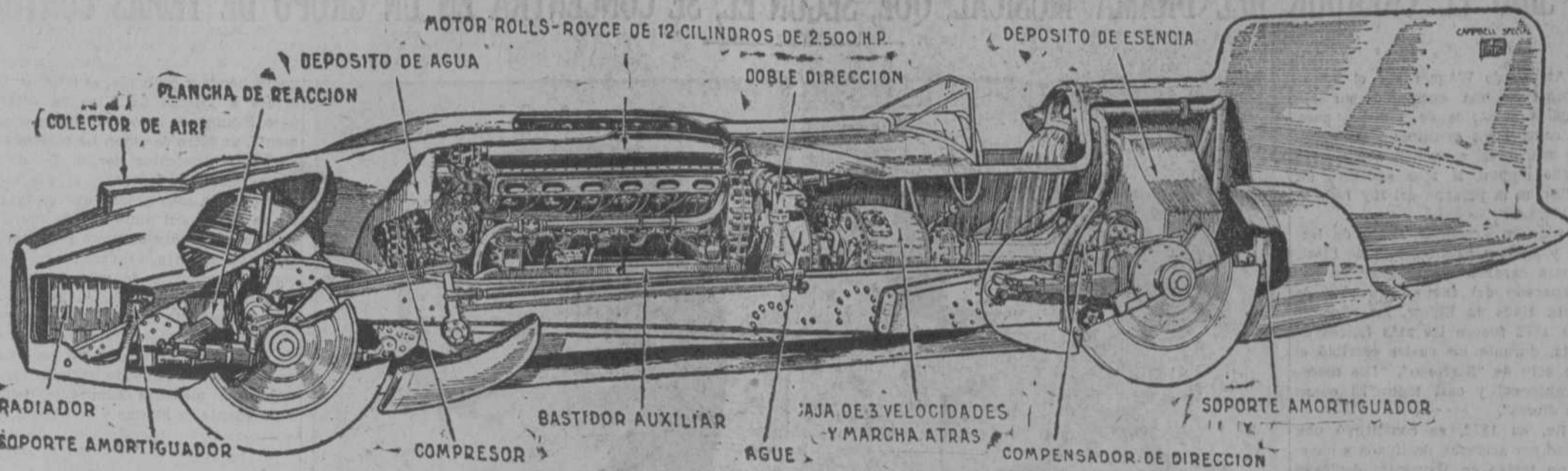
Un corte, dibujado en el estudio técnico de "The Motor", del "Pájaro Azul", con el que Sir Malcolm Campbell intentará alcanzar la fantástica velocidad de 450 kms. por hora.
