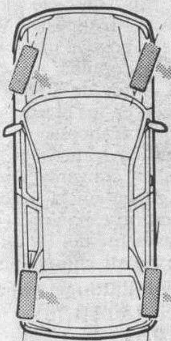
El tren trasero autodireccional es un gran avance para ganar en estabilidad en los terrenos virados. Para ganar en seguridad.
