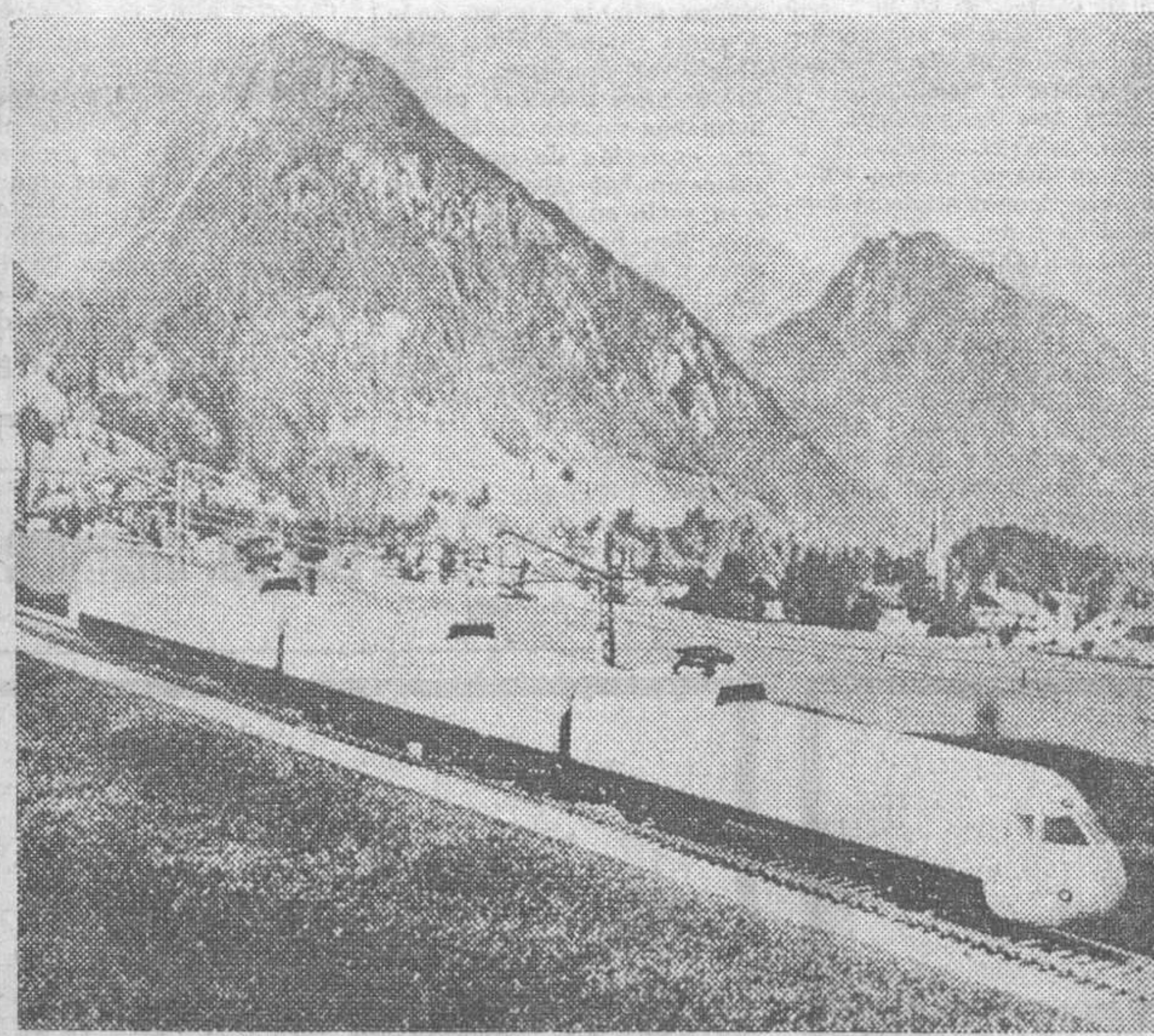
Un nuevo tren de pruebas que podría alcanzar hasta 400 kilómetros por hora de velocidad, está siendo ensayado en la RFA. Las pruebas forman parte de un programa en el que los vehículos que circulan sobre carriles están siendo tecnológicamente actualizados para hacerlos más rentables en su explotación y más adecuados para los tiempos veloces en que vivimos. La foto muestra el citado tren durante las pruebas. — (Foto FIEL).
