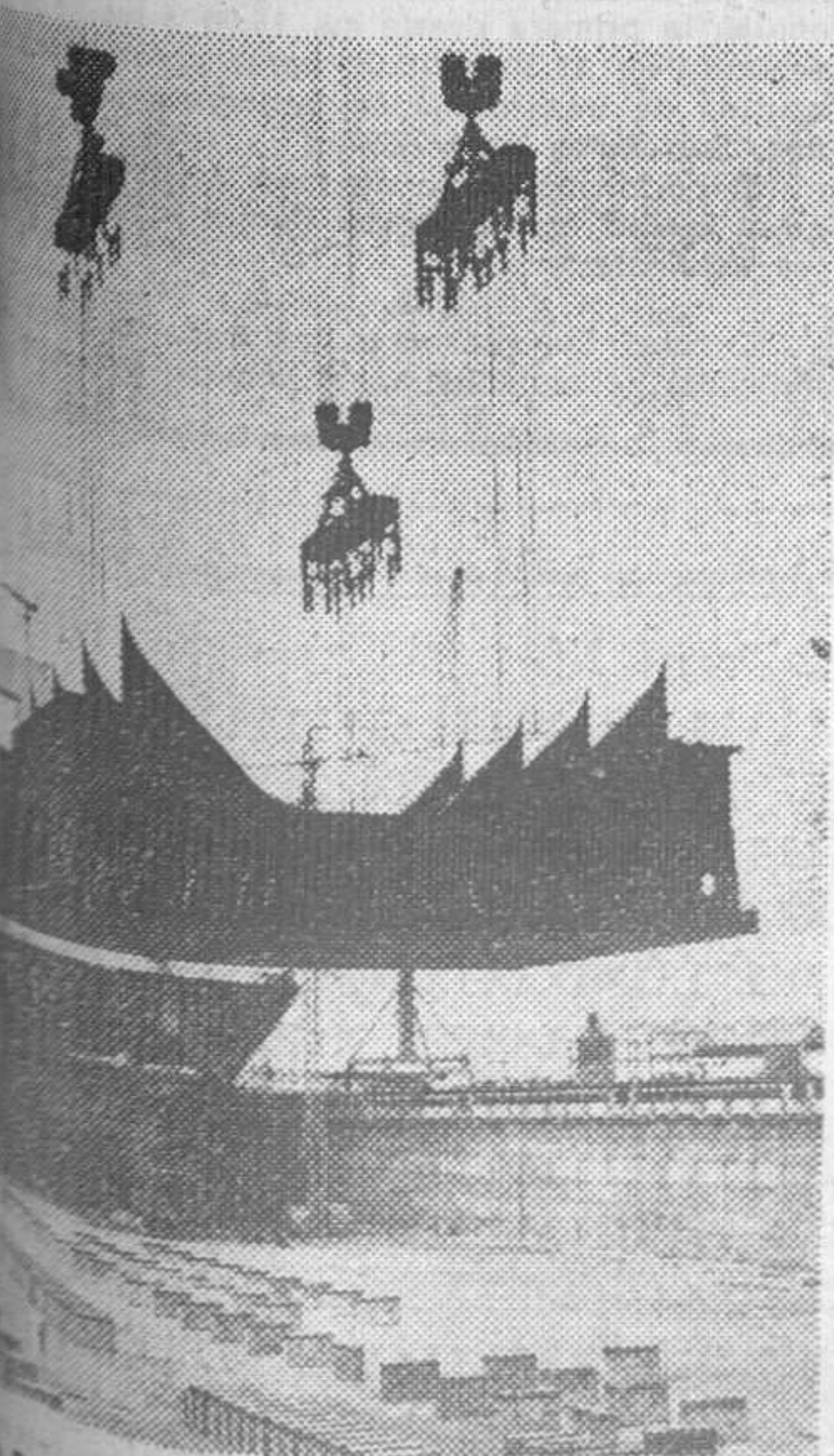
(Cádiz). — Esta gigantesca quilla de 457 toneladas de peso en el momento de ser montada en un petrolero de 260.000 TPM., que se construye en esta factoría de Astilleros Españoles, para una naviera de Santander. — (Foto Cifra).
