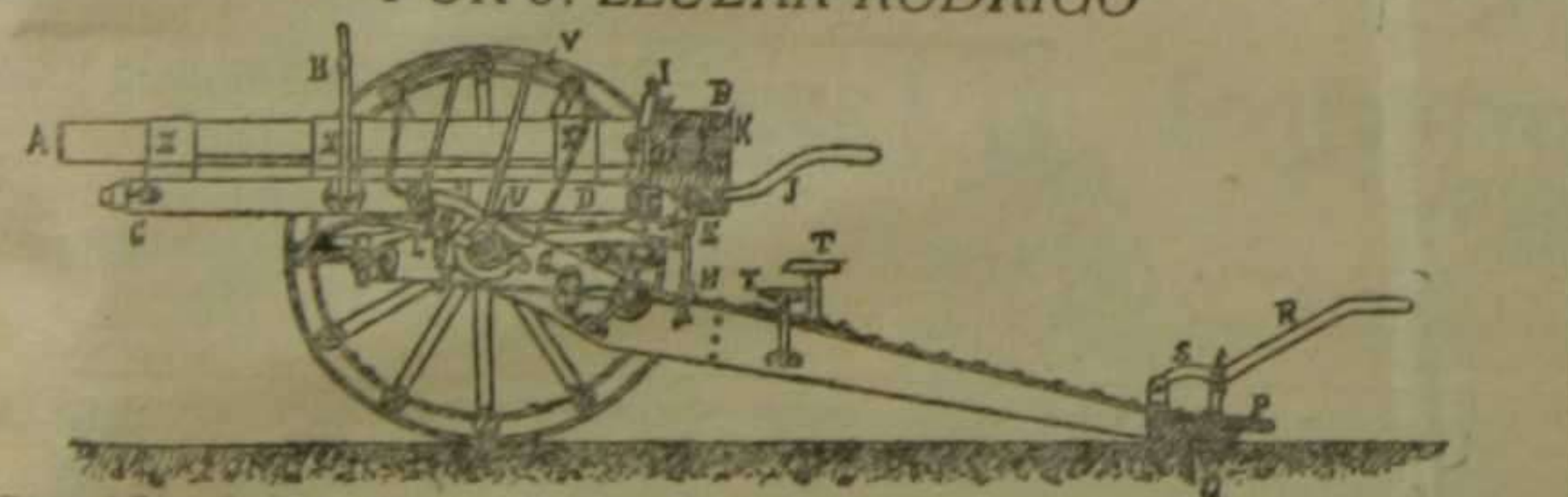
Figura 12.—Pieza Krupp de campaña de tiro rápido, de 96 milímetros, empleada por el ejército alemán. Su mecanismo es análogo al de la novísima pieza de 77 del mismo sistema
