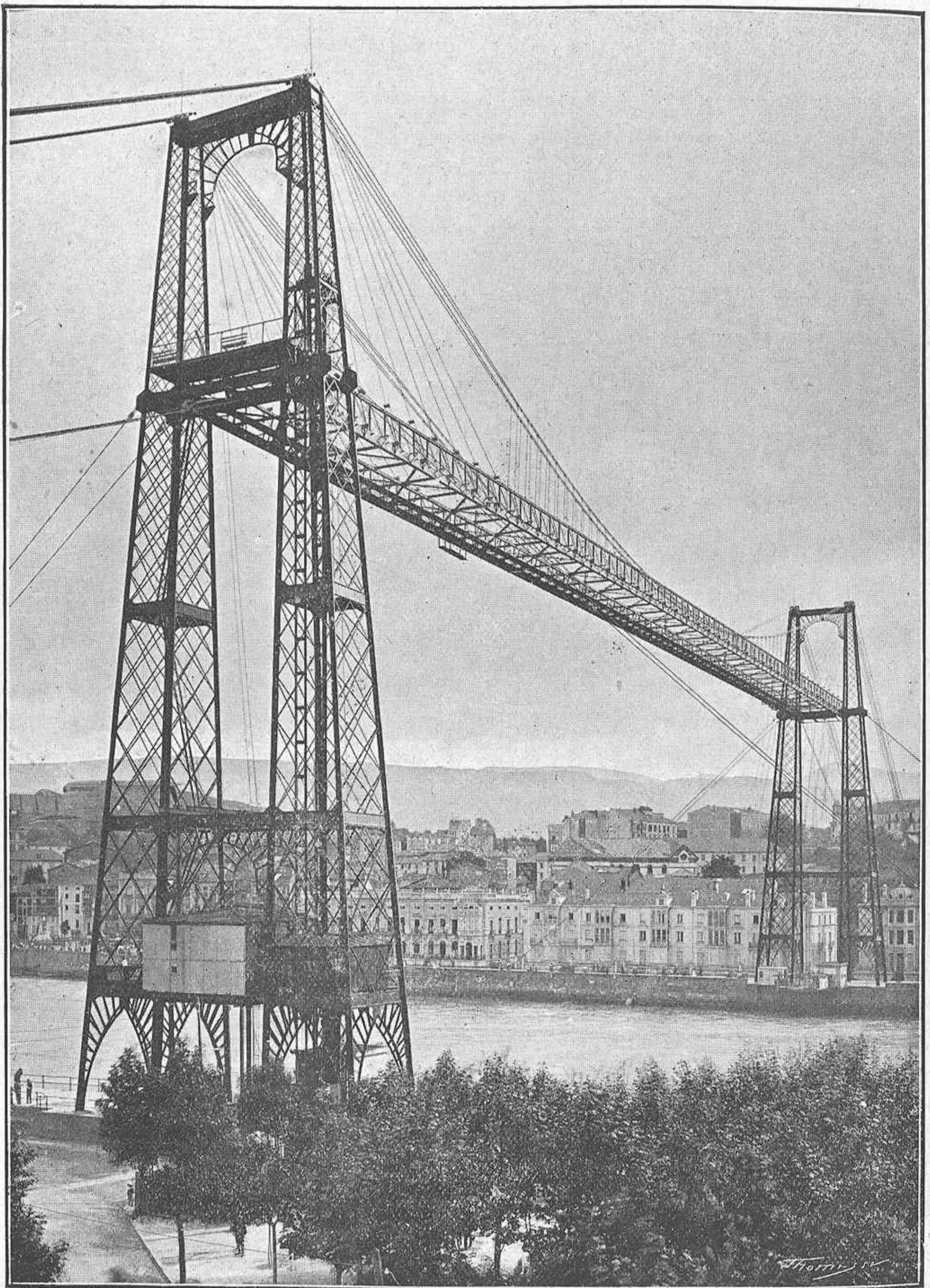
PUENTE «VIZCAYA» ARENAS-PORTUGALETE (BILBAO)
