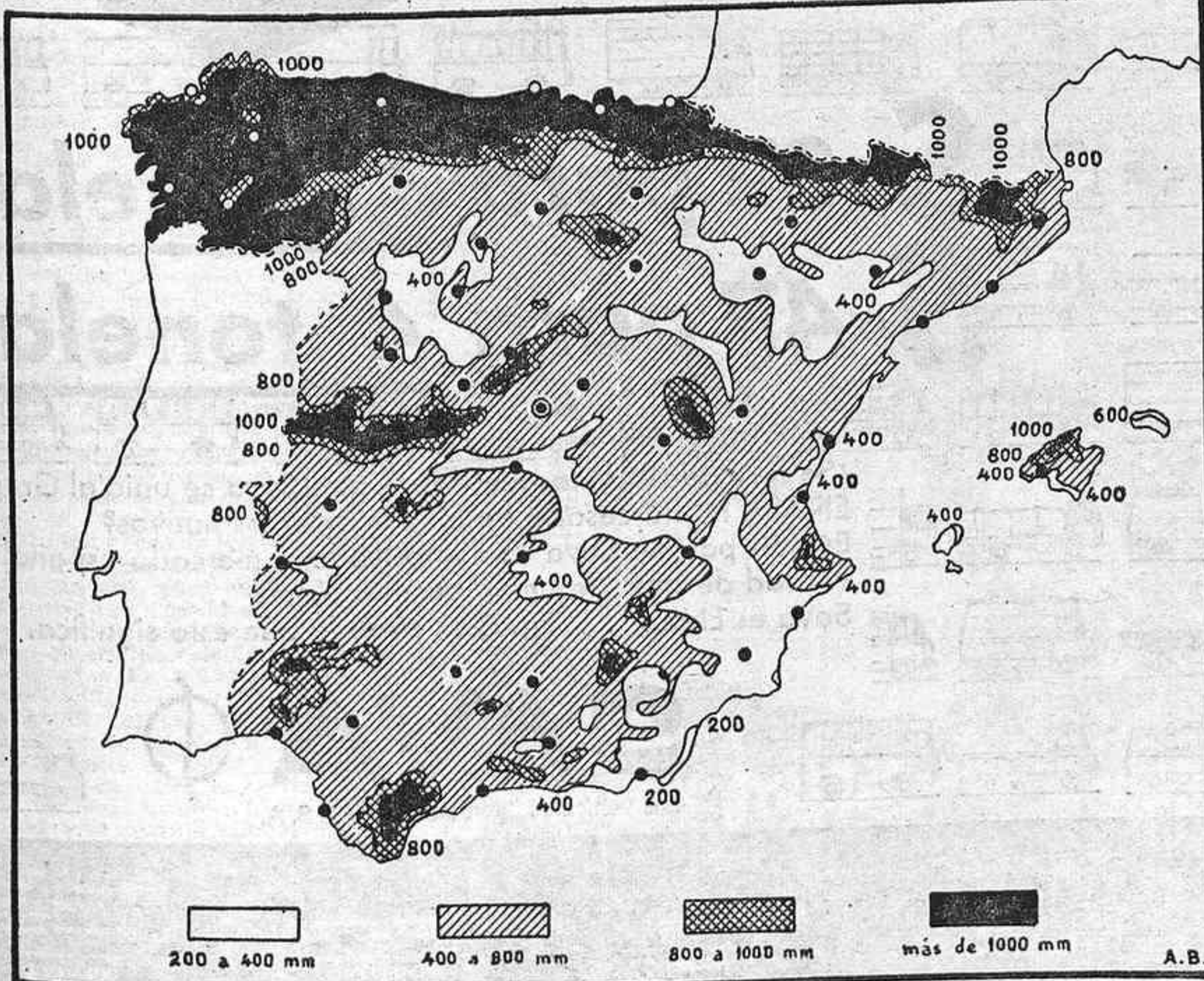
MAPA DE PRECIPITACIONES MEDIAS (1931-60). — Servicio Meteorológico Nacional. Un valioso ejemplo del aprovechamiento y explotación de datos climatológicos es la distribución de las lluvias en España
