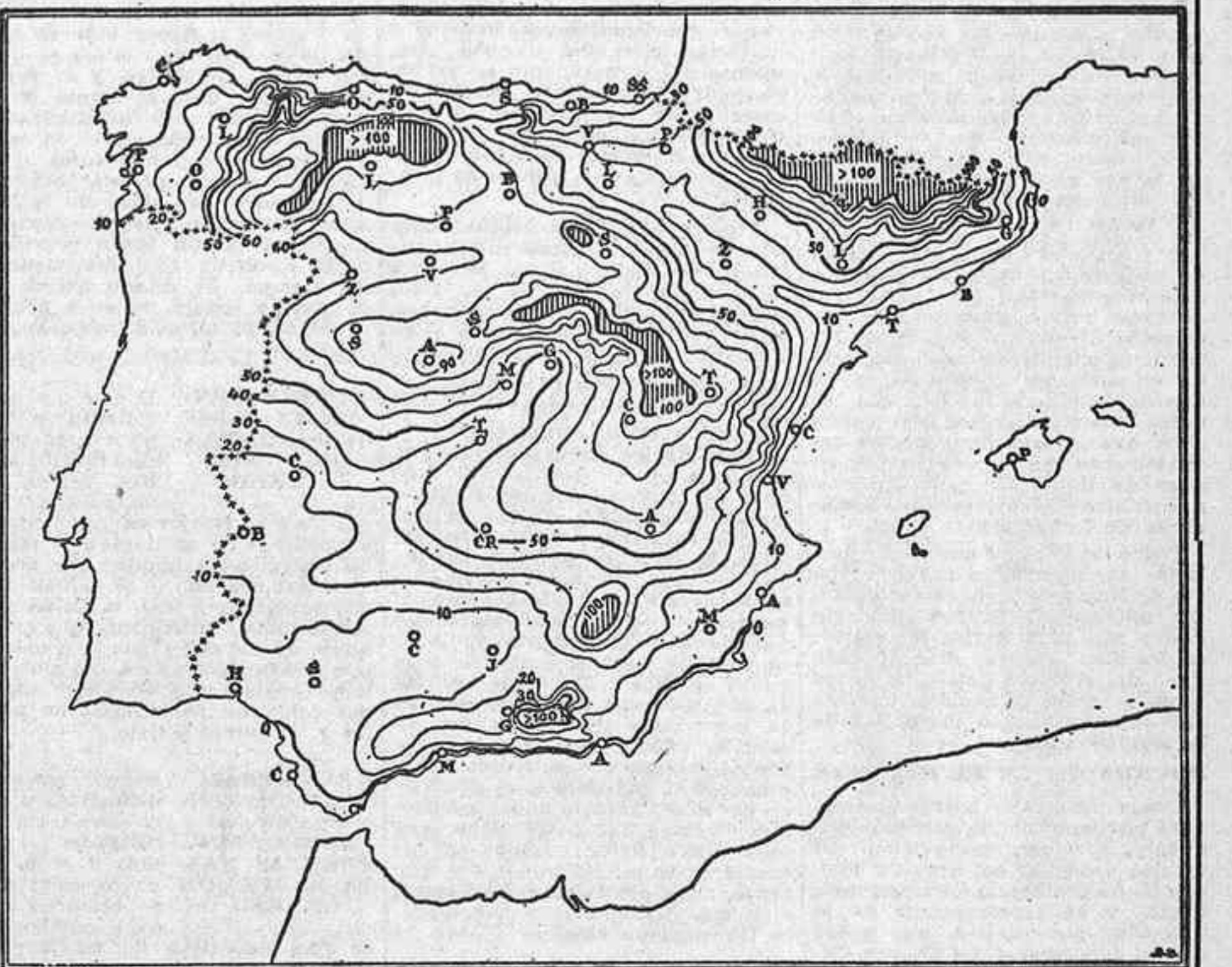
Promedio anual de número de días de helada en España. Obsérvese cómo los "polos de frío" con más de cien días de helada al año aparecen por las montañas de León, Pirineos y cordilleras Central e Ibérica. Madrid tiene una media anual de sesenta días de helada
