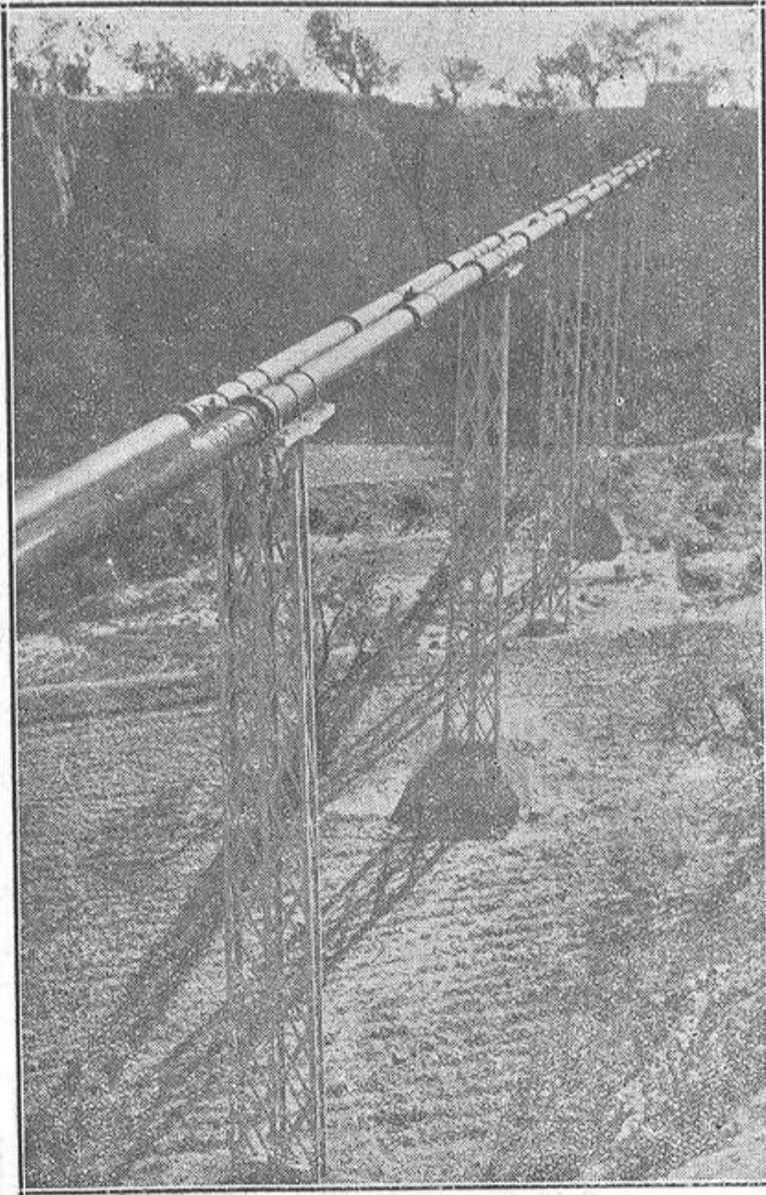
CRUCE DEL BARRANCO DE VERDUNA 2 tuberías de 300 m/m de diámetro, 1928
