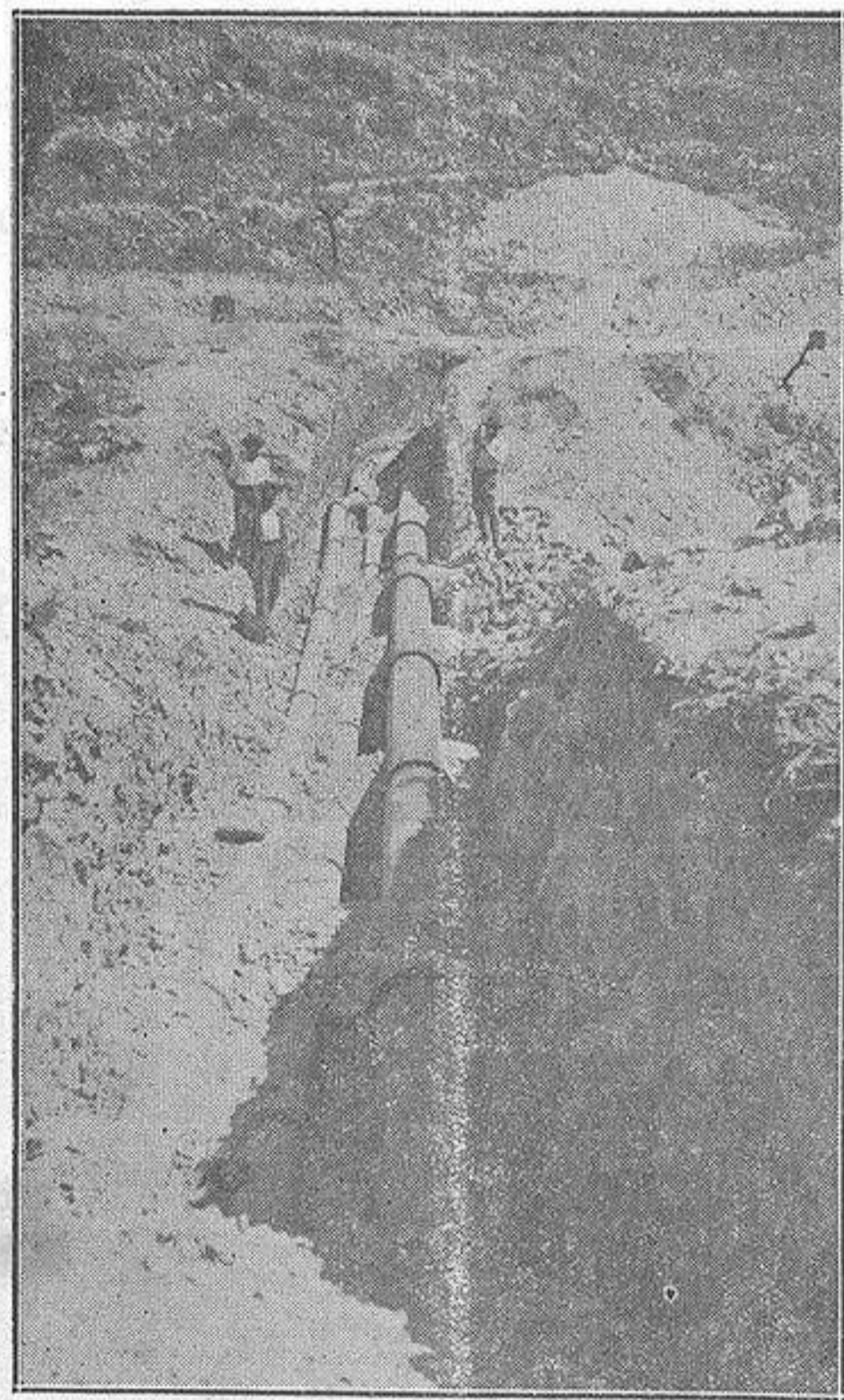
Tuberías colocadas entre Los Calderones de Novelda y el Collado de la Chirichola, 1928
