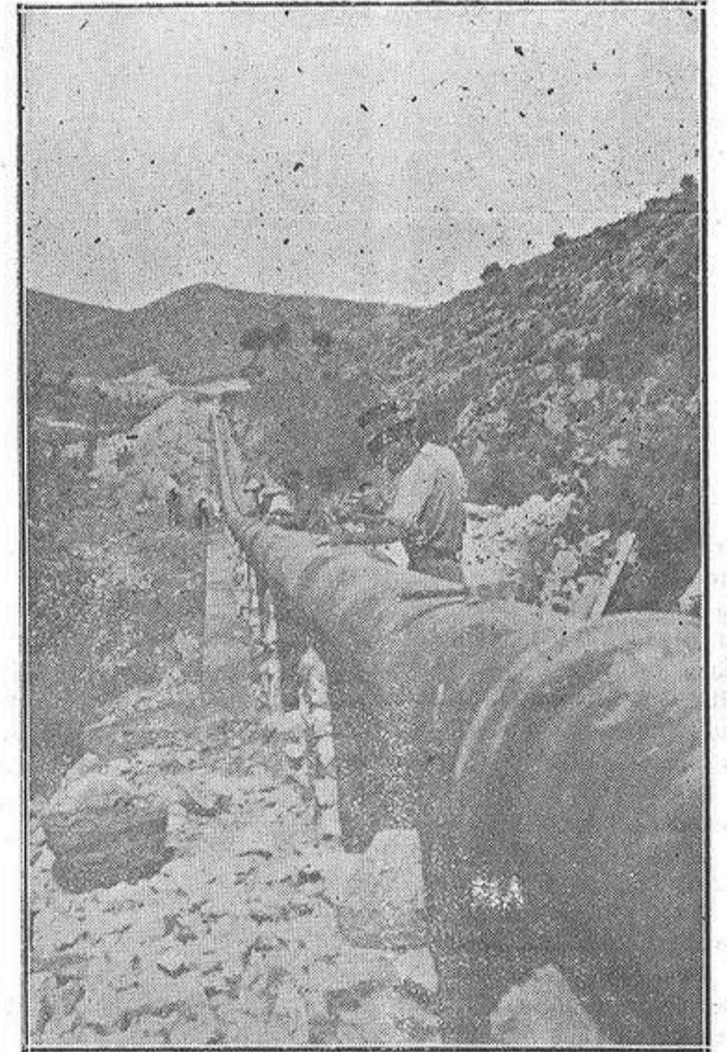
Tuberías de a 400 m/m de diámetro entre los kilómetros 25 y 26. Término de Novelda, 1928
