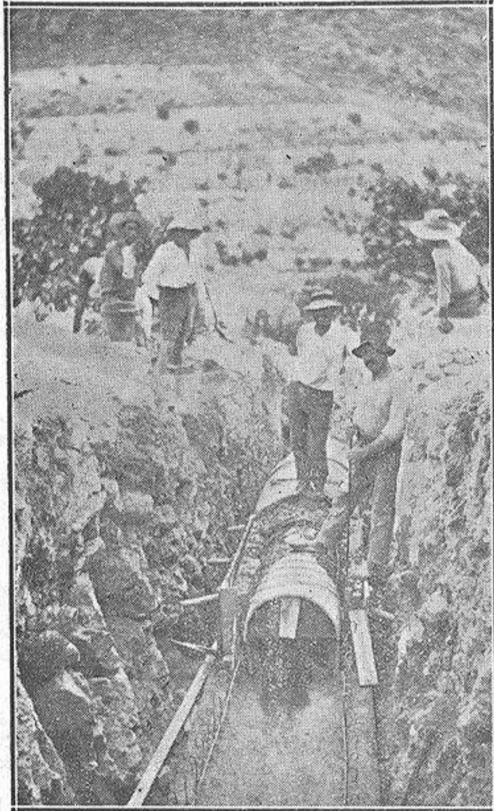
CANAL OVOIDE a la bajada de Los Calderones de Novelda, 1928
