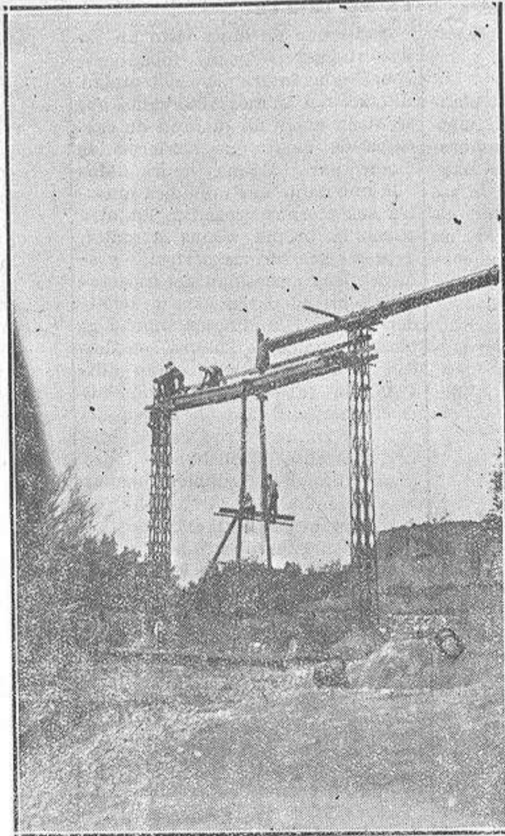
BARRANCO DE VERDUNA Colocación de los tubos, detalle del montaje
