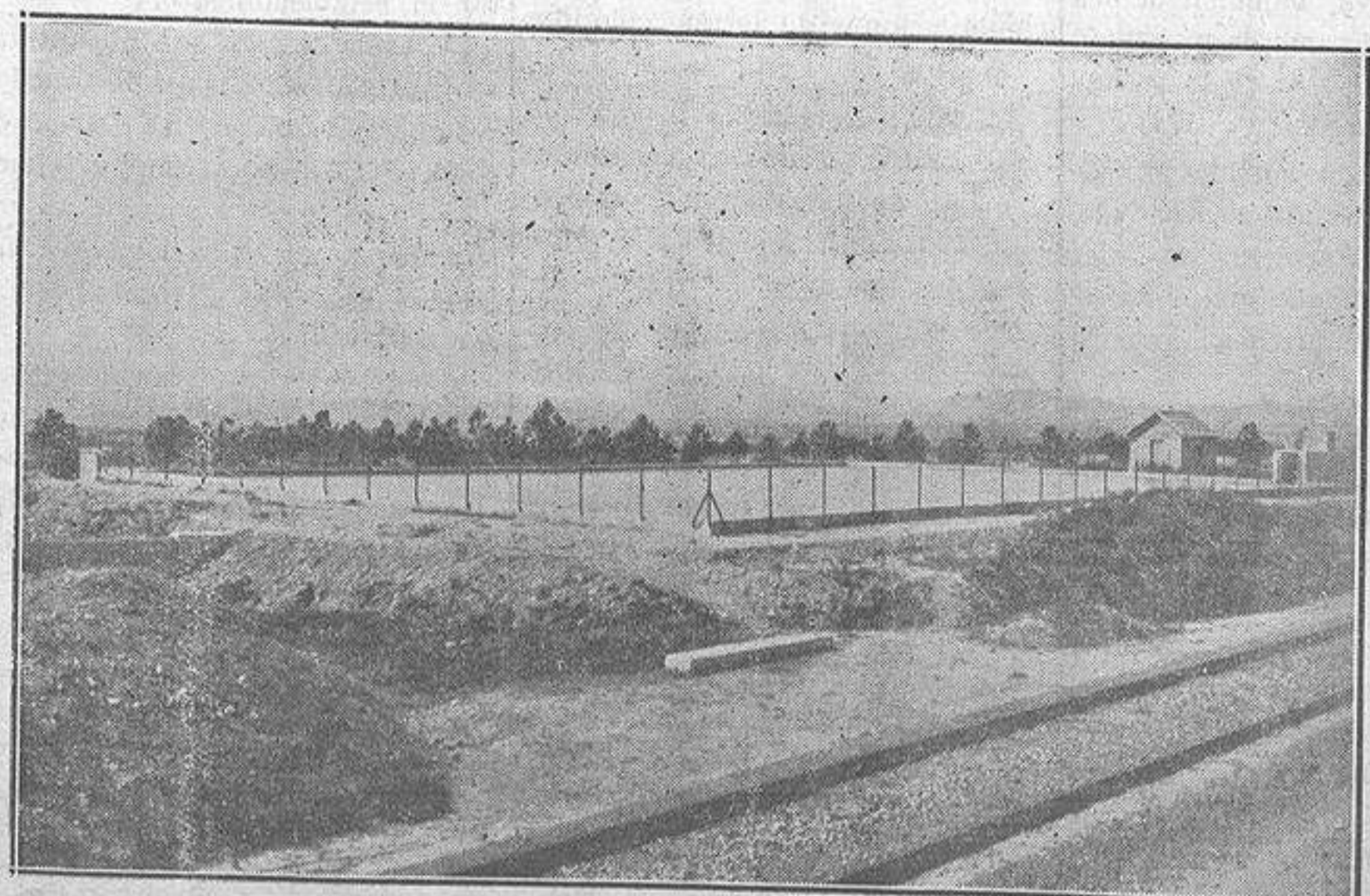
Bolsa de Riegos agrícolas de La Cuba de Monforte del Cid 4.500 metros cúbicos de cabida, 1929.
