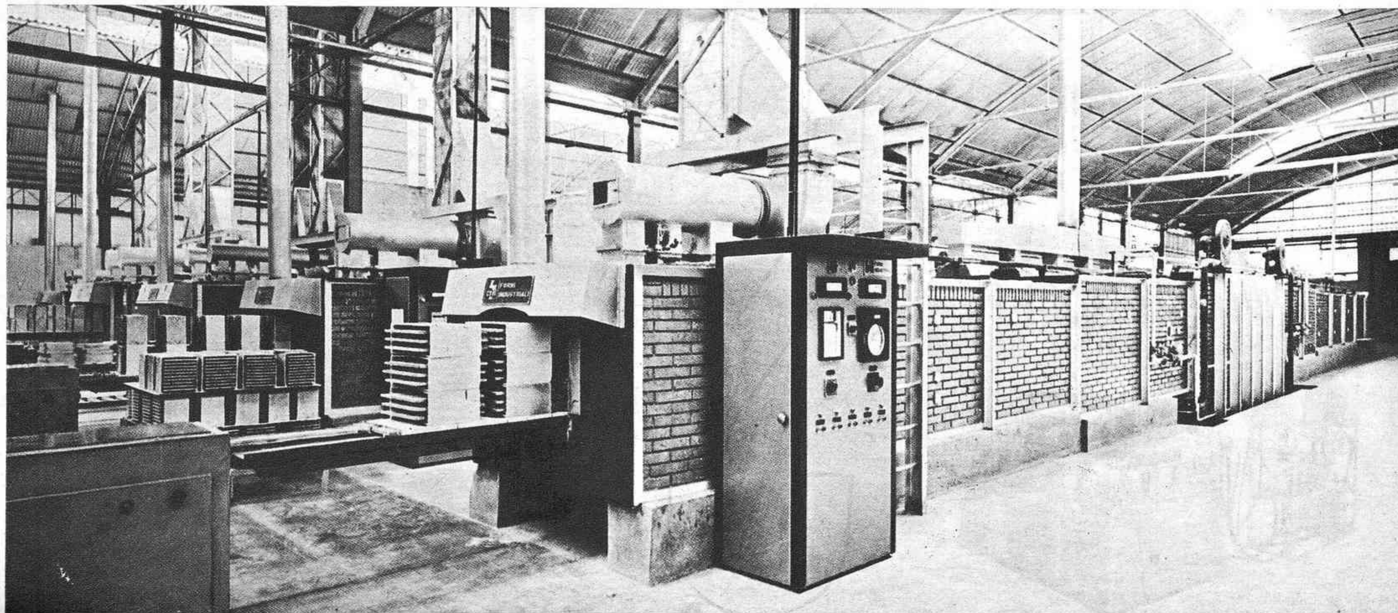
Hornos bicanales para esmaltados
