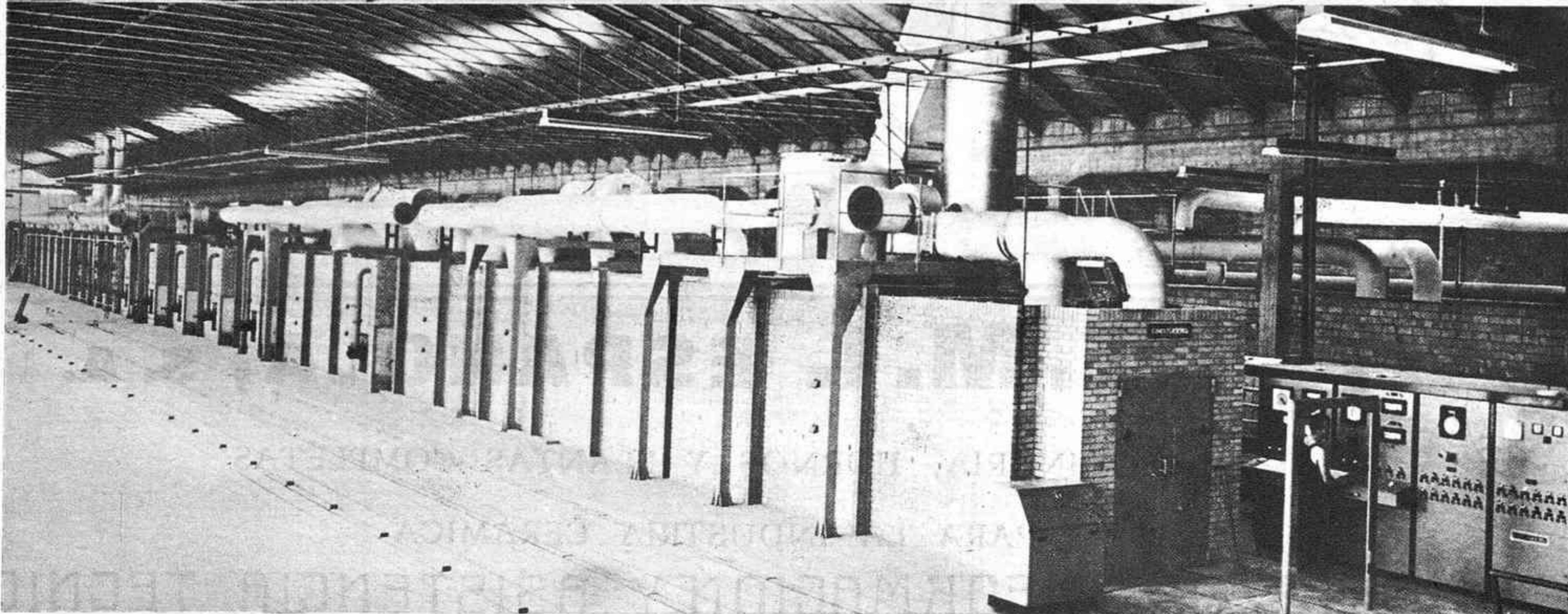
Hornos tuneles para biscochado y esmaltado
