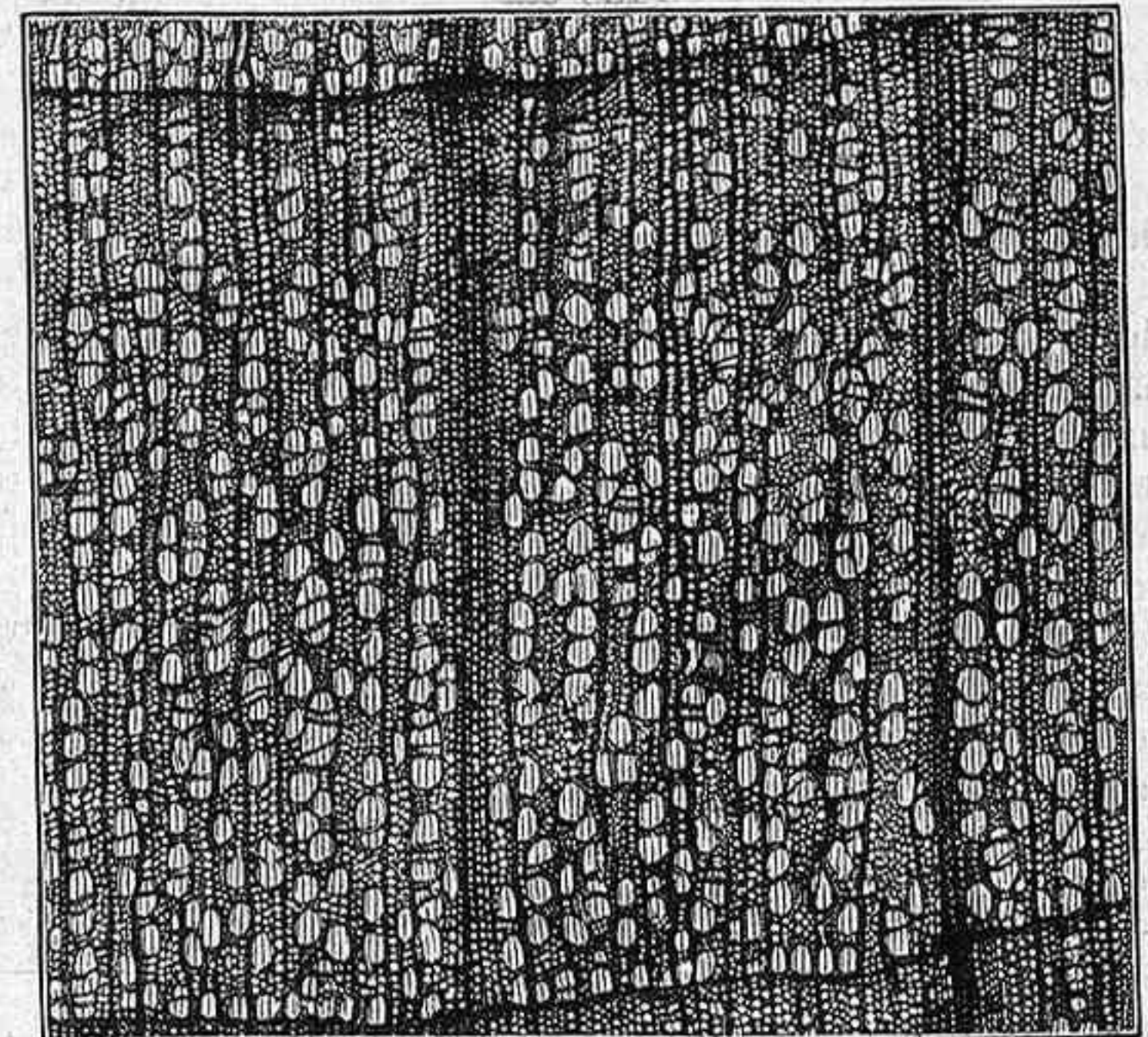
Fig. 3. - Aliso blanco ( Alnus incana , D.G.). - Sección transversal. Aumento 30 diámetros.
