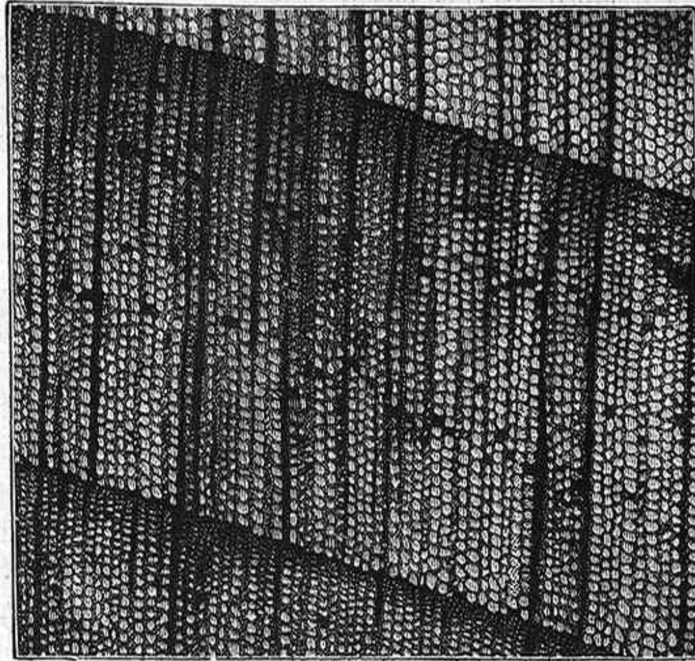
Fig. 2. - Enebro de Fenicia ( Juniperus Phoenicea , Linn.). Sección transversal. - Otro tipo de la misma madera sin canales resiníferos. La resina está encerrada en algunas fibras que se destacan por su color negro. Aumento 60 diámetros.
