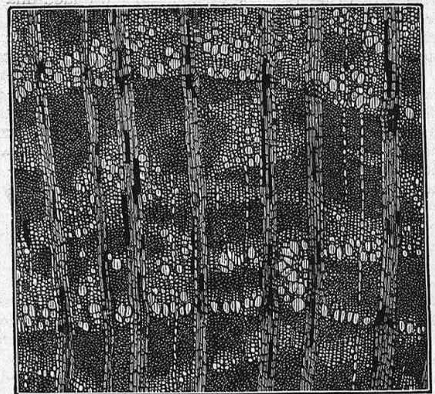
Fig. 6. - Aulaga de Europa ( Ulex europaeus , Linn.) Sección transversal. Aumento 30 diámetros.
