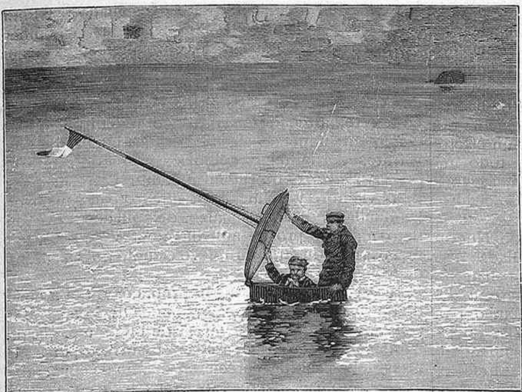
Fig. 1. - Prueba del submarino Goubet practicada en Cherburgo en 1.º de febrero de 1890. El Goubet cerrando su porta. (De una fotografía.)
