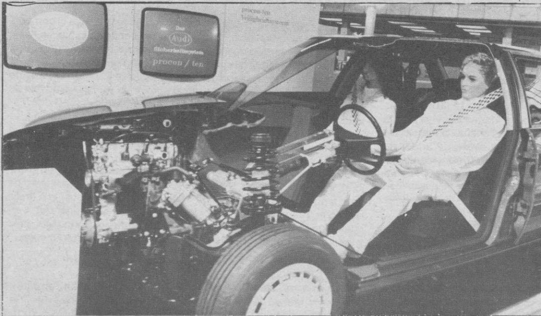
Sección de la parte delantera de un coche que incorpora el sistema de seguridad «Procon-Ten», donde se puede apreciar el cable sujeto al volante y al cinturón de seguridad del conductor
