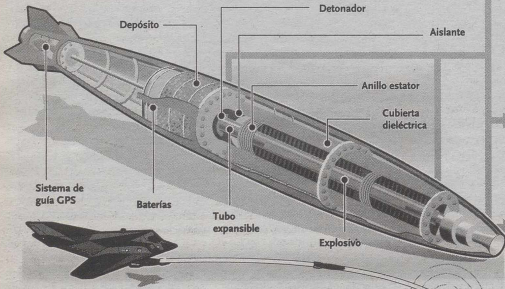
A. Una corriente del detonador llega al estator y crea un campo magnético. La explosión expande el tubo
