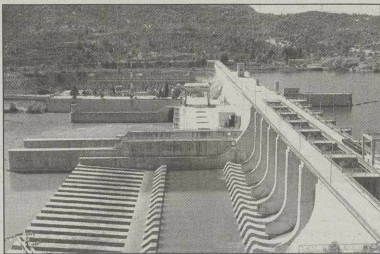
Embalse de Ribarroja, sobre el río Ebro.
