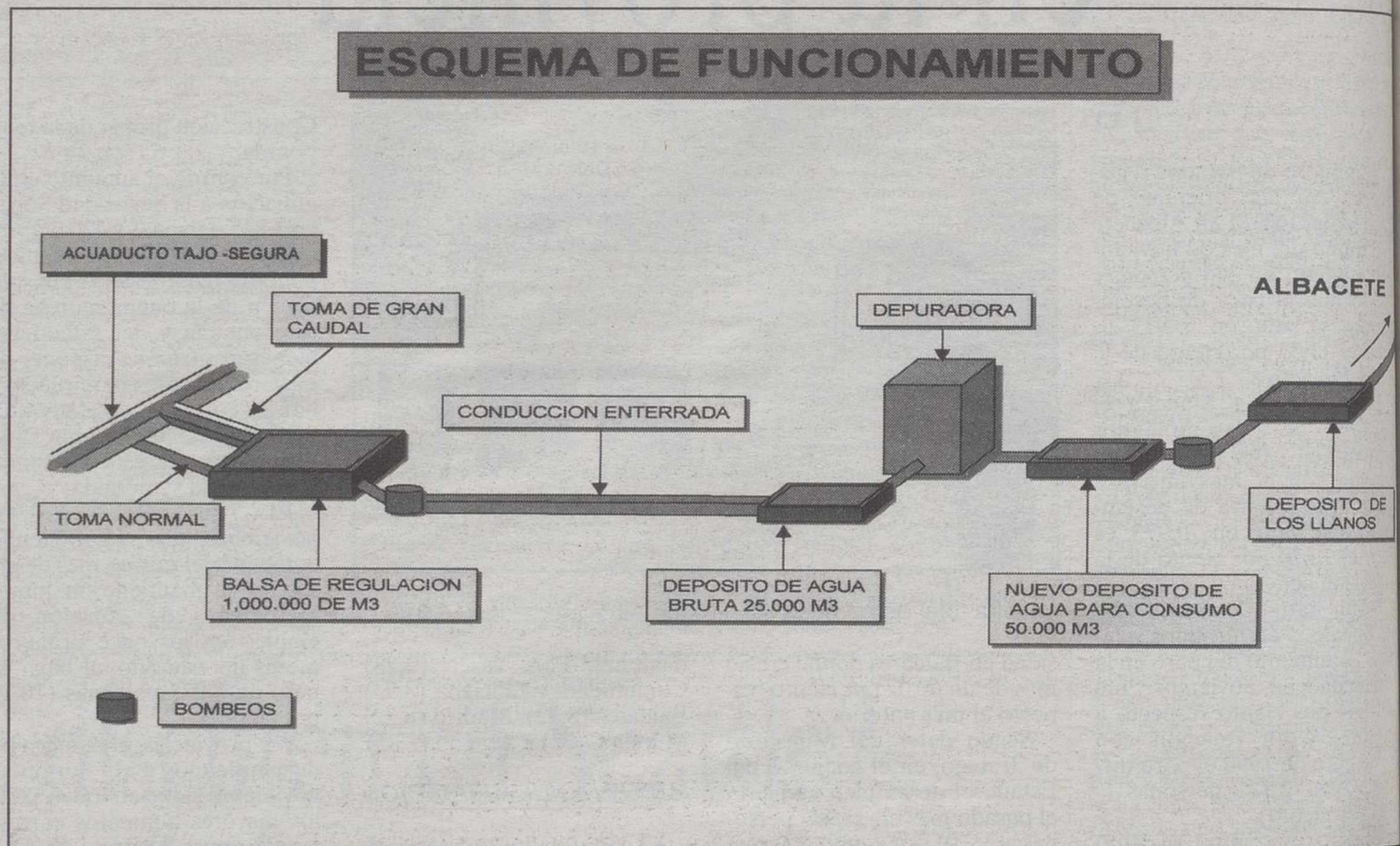
Esquema de funcionamiento del proyecto para el nuevo suministro de agua de Albacete.
