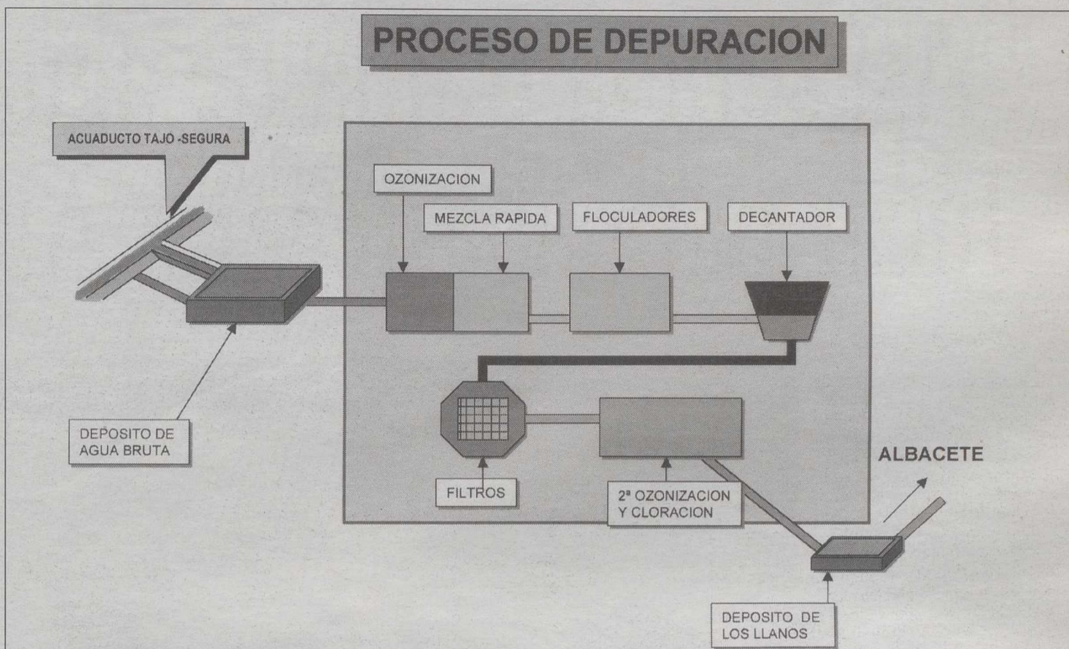
Esquema general del funcionamiento de la futura depuradora.
