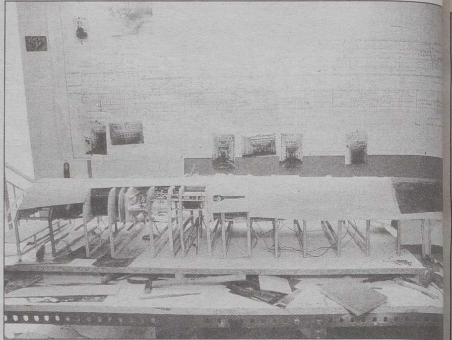
El director de factoría de Unión Naval Valencia facilitó los planos para construir el barco.
