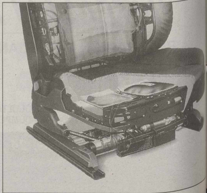
El asiento activo de BMW.
