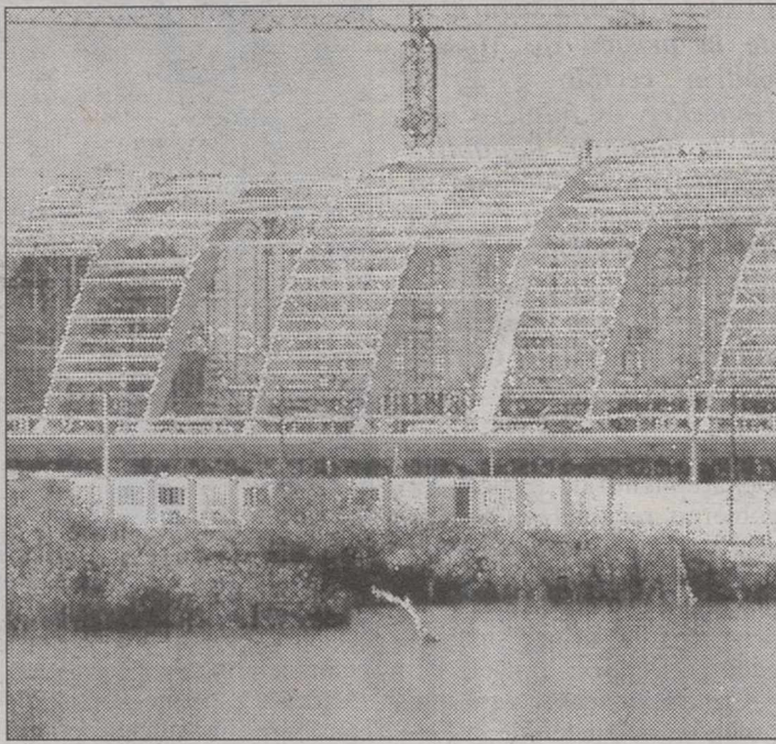
Aspecto general de las obras al borde de la dársena del Guadalquivir.
