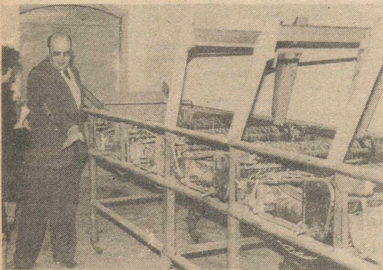
Maquina que está destinada a seleccionar los ajos para clasificarlos en las distintas categorías.
