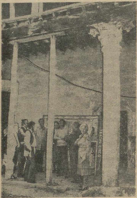
Las vigas, apuntaladas.
