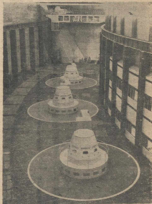
Valdecañas.—Interior central. Potencia, 225.000 kw.
