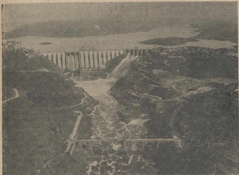
ALCANTARA.—Presa y embalse. Capacidad, 3.162 millones de m 3 .
