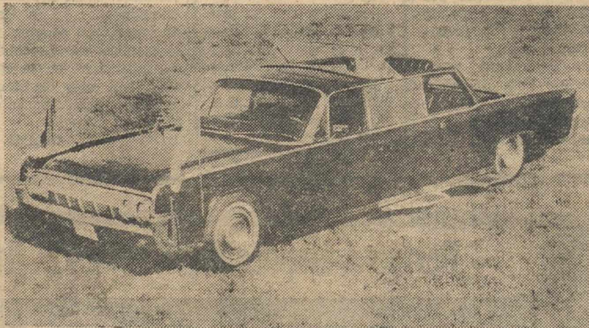
NUEVA YORK.—El Papa Paulo VI usará este automóvil, negro, de veinte pies de longitud, construido por la Lincoln, preparado para cuando el Sumo Pontífice asista al Congreso Eucarístico en Bogotá. El coche tiene un asiento posterior en forma de trono, que puede ser elevado para proporcionar la visión del Papa en los desfiles. Una pantalla de plexiglas resguarda al Pontífice. Las banderas del Vaticano y Colombia están a ambos lados del automóvil, en su parte delantera. (Telefoto UPI-CIFRA).
