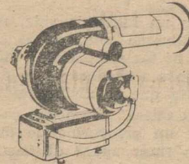
QUEMADORES AUTOMATICOS THERMEX Tipos FJ y FI Potencia calorífica: 12.000 a 100.000 Cal/H. Combustible: Petróleo o Gas-Oil Pulverización: Mecánica
