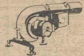
QUEMADORES AUTOMATICOS THERMEX Tipos D-2, D-3, D-4, D-5 y D-6 Potencia calorífica: 75.000 a 2.000.000 Cal/H. Combustible: Petróleo o Gas-Oil Pulverización: Mecánica
