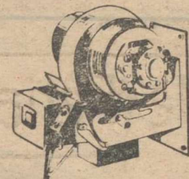
QUEMADORES AUTOMATICOS THERMEX Tipos T-1, T-2, T-3 y T-4 Potencia calorífica: 16.000 a 165.000 Cal/H. Combustible: Petróleo o Gas-Oil Pulverización: Mecánica
