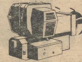
QUEMADORES AUTOMATICOS JOANNES Tipos JS-10, 20, 35, 50, 80, 100 y 150 Potencia Calorífica: 50.000 a 1.200.000 Cal/H. Combustible: Fuel-Oil Pulverización: Mecánica
