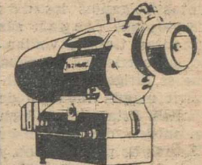
QUEMADORES AUTOMATICOS JOANNES Tipos SUPER G-7, G-12, G-23, G-35, G-45 y G-50 Potencia calorífica: 16.000 a 480.000 Cal/H. Combustible: Fuel-Oil Pulverización: Neumática
