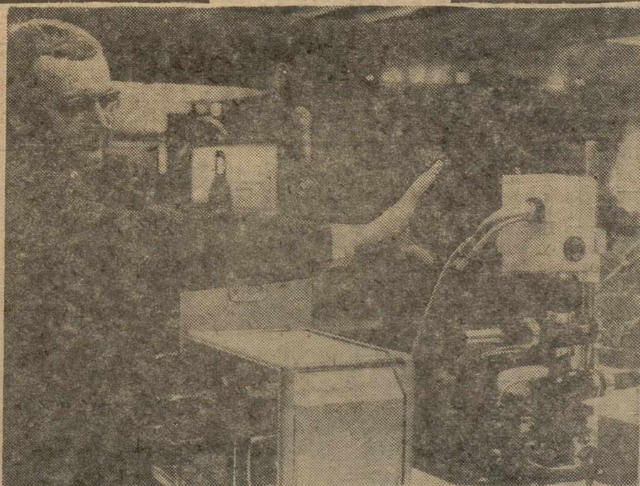
He aquí un aparato Laser fabricado por la industria Carl Zeiss de Jena (Alemania del Este), mediante el cual puede hacerse visible por un microscopio la millonésima parte de un milímetro. Forma parte del material expuesto en el Certamen Internacional de Düsseldorf para la automatización y la técnica de la medida.—(FOTO FIEL).
