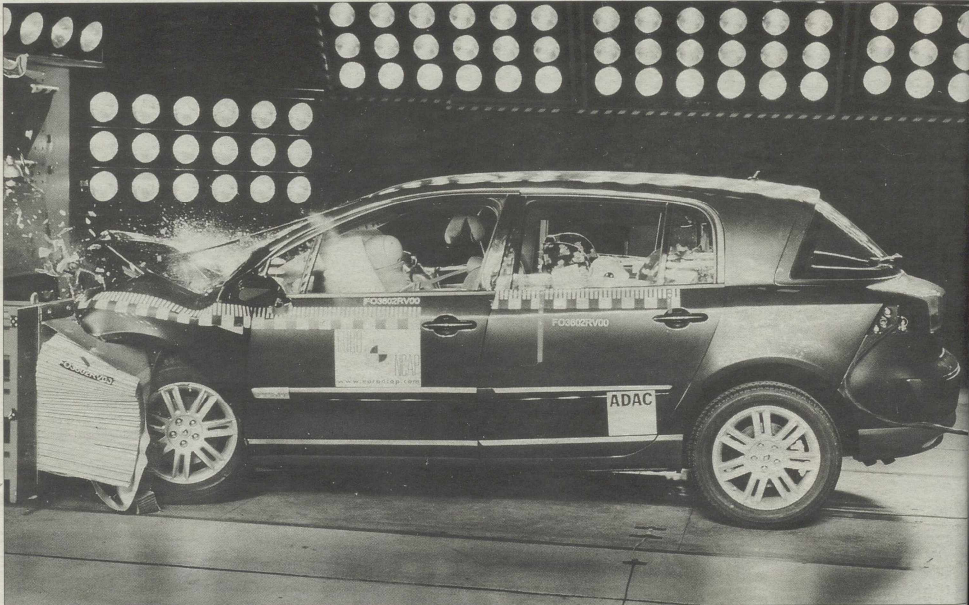
Imagen de la prueba de colisión frontal realizada al Renault Vel Satis, que obtuvo 5 estrellas en seguridad. En la foto inferior, muñecos de niños sirven para analizar cómo afectan las colisiones a éstos.
