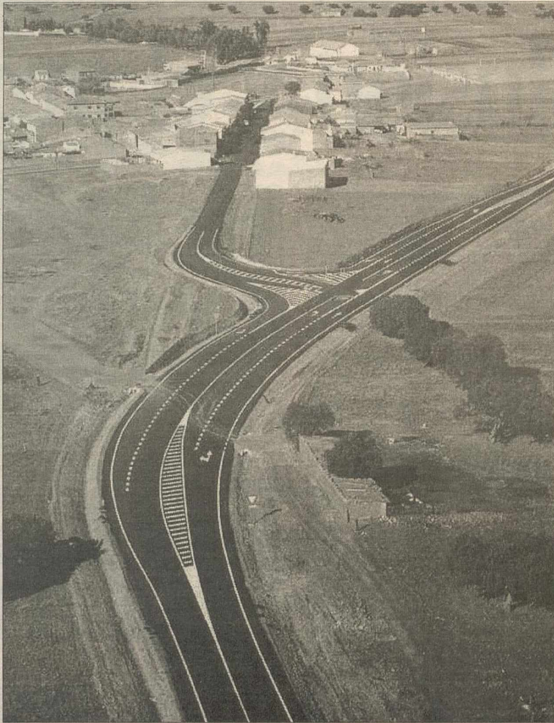
Vista aérea de la intersección y variante de Saceruela (ya finalizada).
