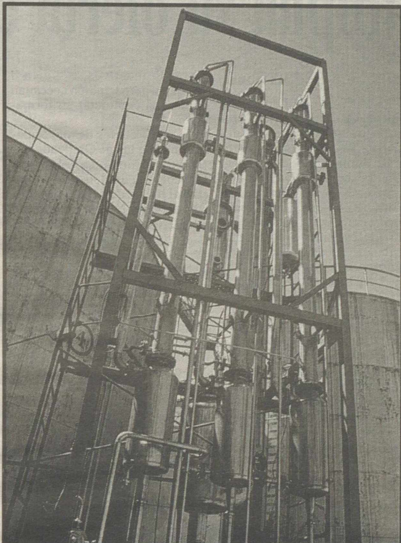
Planta experimental de concentración de alpechín.
