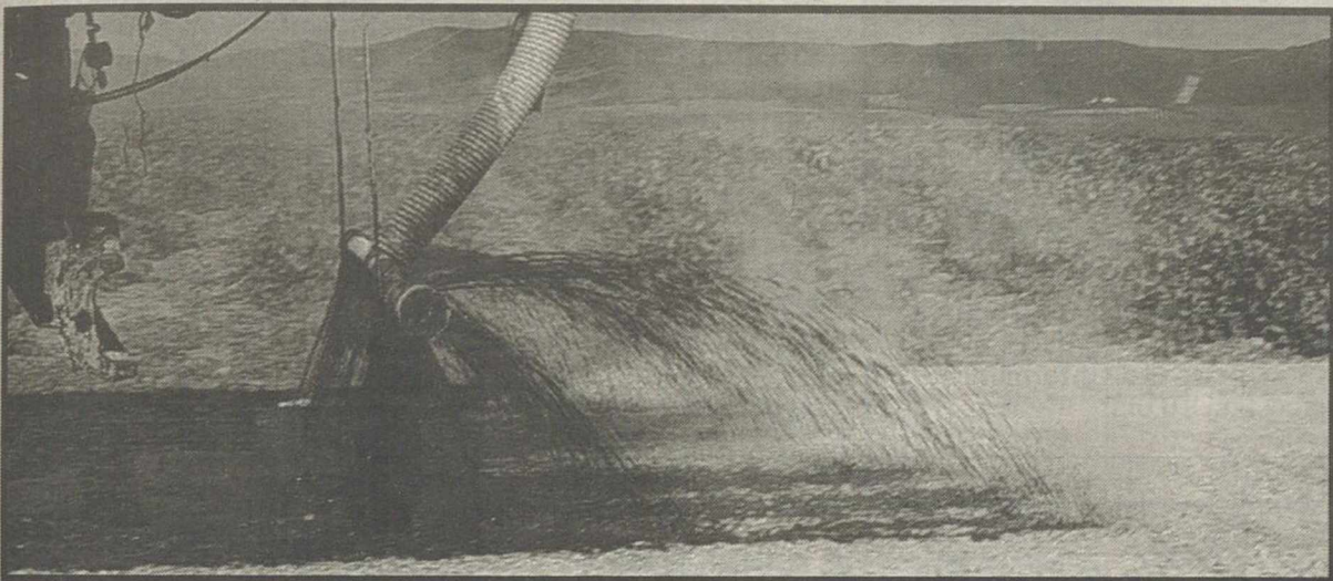
Extensión de alpechín sobre la mezcla de suelo y cal.
