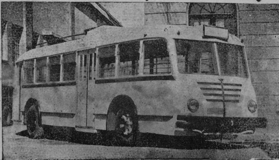
La Sociedad General de Tranvías Eléctricos Interurbanos de Palma, ha adquirido seis autobuses Hispano-Suiza para mejora de sus servicios. Tienen 9'300 metros de largo y 2'480 de ancho. Su cabida es de 25 pasajeros sentados y 45 de pie. Su marcha máxima es de 70 kms. hora. Llevan seis marchas y dispositivo de retroceso que garantiza su seguridad en las paradas en cuesta.
