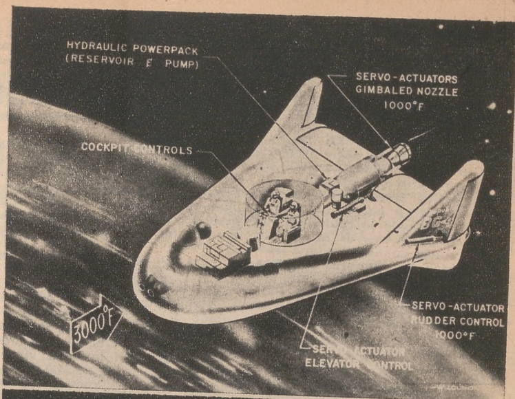
Proyecto de construcción de una estación del espacio, base de naves espaciales
