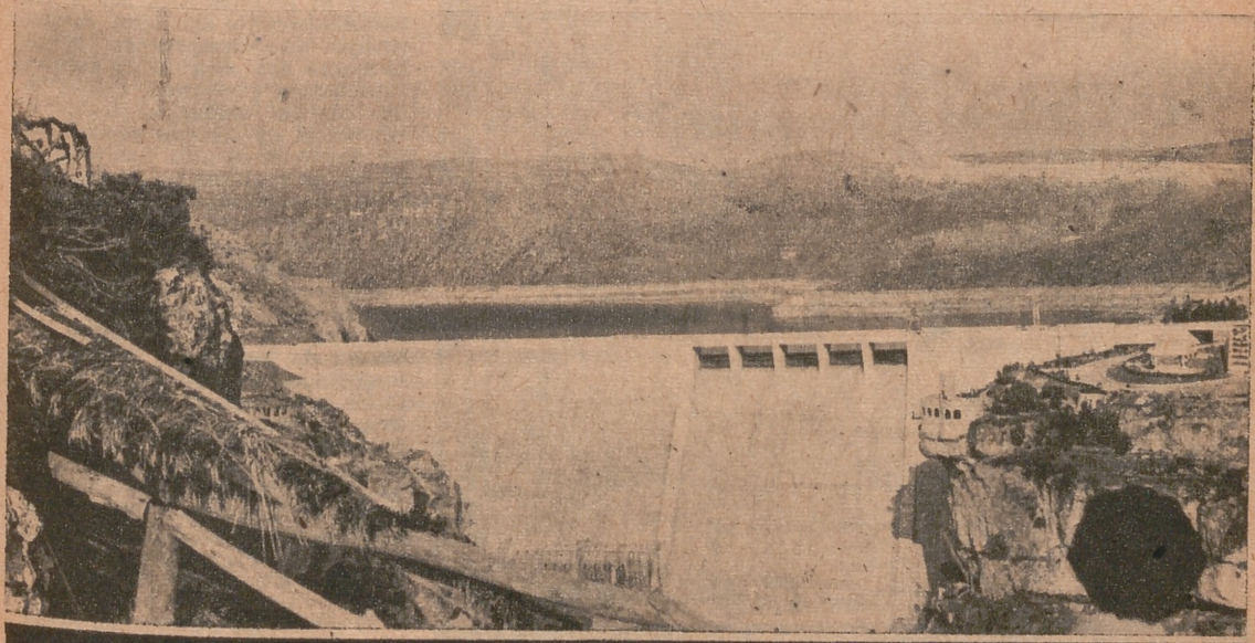
El pantano de Entrepeñas, una de las últimas realizaciones energéticas
