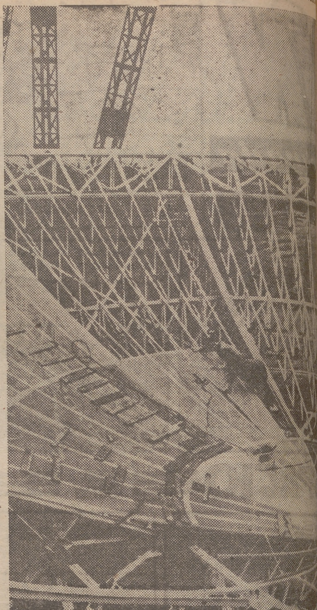
Un nuevo telescopio gigante está en construcción en la República Federal Alemana cerca de Munster. El diámetro del radar cóncavo mide 25 metros. En la foto, mecánicos de la fábrica Zeppelin, de Friedrichshafen, trabajan en el nuevo telescopio gigante. (Foto Keystone Nemes)
