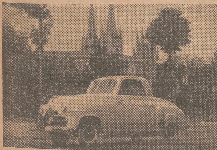
He aquí el automóvil nacional 'Kapi', construido en Burgos, por el capitán don Federico Saldaña. Tiene una potencia de dos caballos y medio y puede desarrollar una velocidad de 75 kilómetros por hora, con un consumo de gasolina de 3,75 litros por 100 kilómetros. (Foto Cifra Gráfica)
