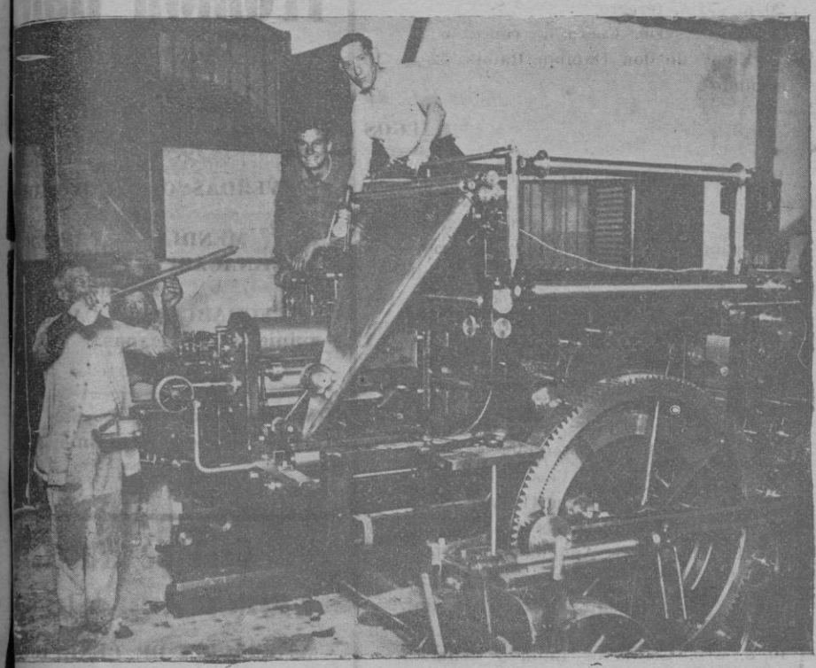
El montaje de la rotoplana "Duplex" en nuestros talleres, para imprimir de mayor tamaño LA ALMUDAINA Fot. Vila
