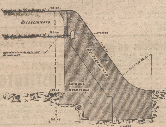
Ataguía de aguas arriba, después del recrecimiento
