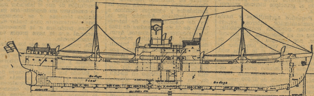
Corte longitudinal del modelo de los barcos que para la flota frutera construye actualmente COFRUNA
