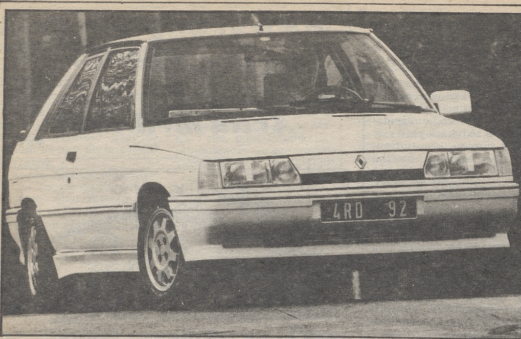
Vehículo experimental de cuatro ruedas directrices, basado en el Renault 11.
