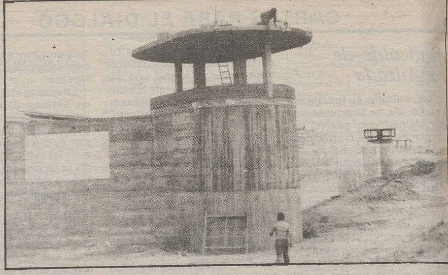
Los muros son de hormigón armado y con una altura de 5,8 metros.
