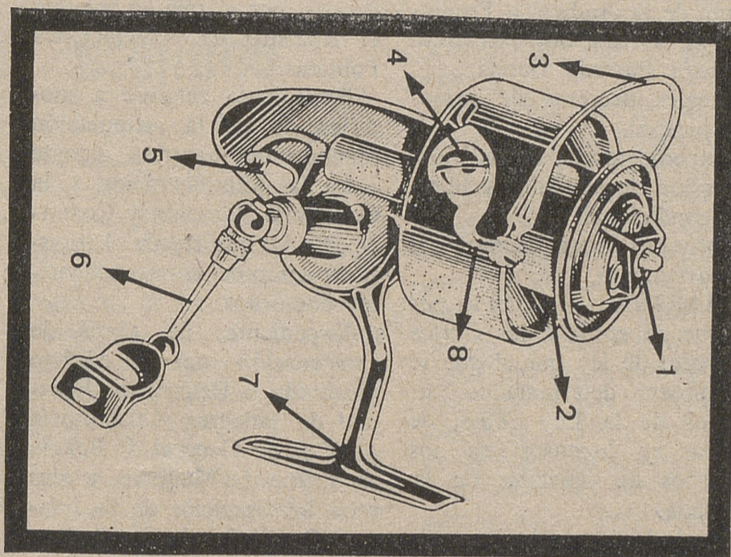
DESCRIPCION DEL CARRETE DE LANCE. — 1. Freno de la fricción. 2. Bobina para envolver el hilo. 3. Arco. 4. Mecanismo del escape del arco. 5. Leva para el frenado silencioso y antirretorno. 6. Manivela. 7. Soporte. 8. Curva para envolver el hilo en la bobina.
