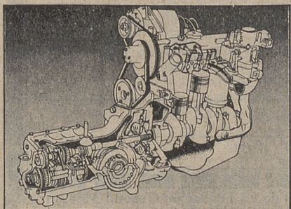
Motor: cigüeñal de 5 apoyos, camisas intercambiables en cilindros, válvulas en cabeza.
