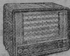
VERTOR (Modelo Temba) 9 lámparas de acción múltiple. Altavoz de 12 pulgadas tipo pesado de alta fidelidad, sistema de bajo a push-pull con 18 vatios de salida (6 veces lo normal) P. v. p. 5.255 — Ptas.
