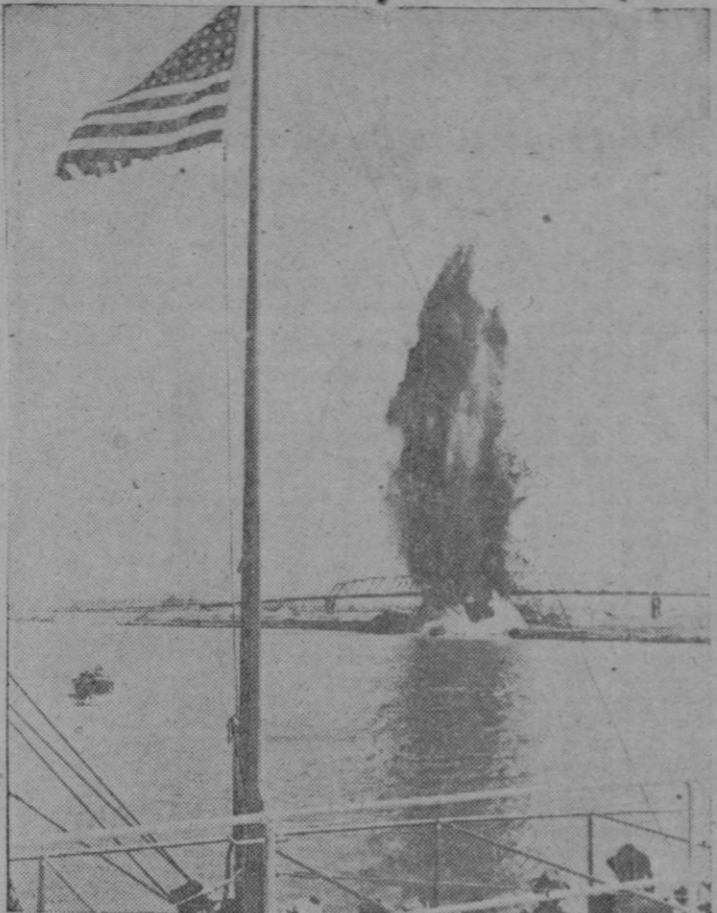
La curva fluvial llamada "Liberty Bend" cerca de Courtney (Estados Unidos), es volada por medio de 326 kilogramos de dinamita con objeto de evitar las inundaciones anuales del río Misuri. Miles de personas presenciaron la explosión desde las orillas y desde un puente recientemente construido.
