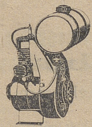
motor refrigerado por aire de 1, 2 y 4 c.v.
