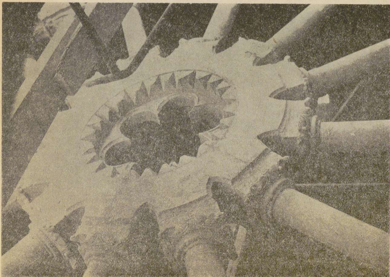
He aquí el centro del sistema radial totalmente substituído con moldeado de cemento. Las líneas de moldeo y de compresión se aprecian perfectamente en la fotografía.
