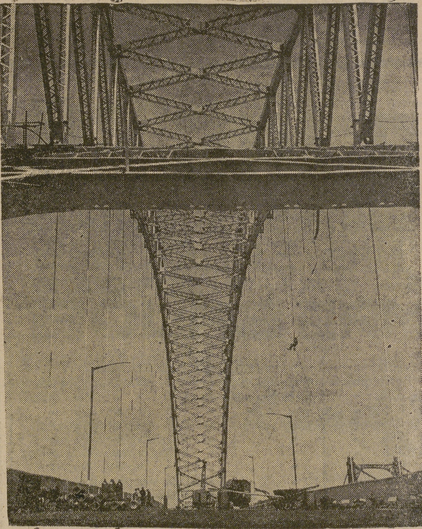
Formando una destacada silueta contra el cielo, puede verse parte de la obra de acero para un puente carretero, valorado en 3 millones de libras, que atravesará el río Mersey
