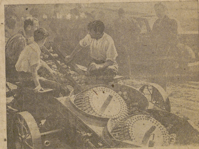
Esta máquina saca las patatas del suelo y las mete en los sacos. Consiste en dos partes. Una que saca las patatas de la tierra y la otra que las clasifica y las mete en sacos o en el remolque. (Calpa)
