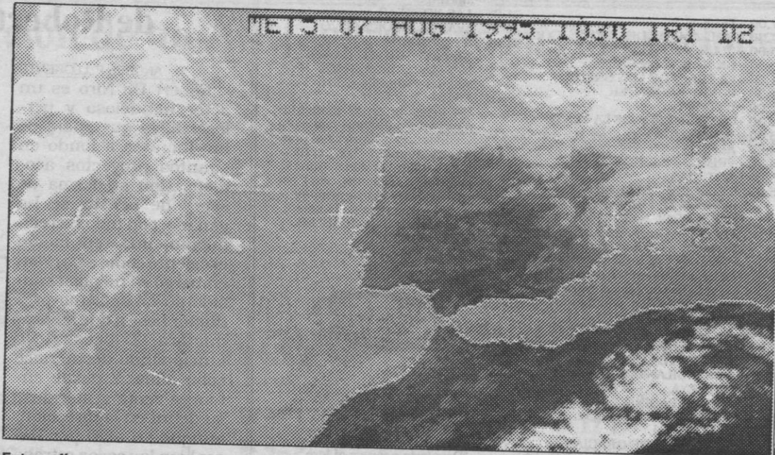
Fotografía tomada por el satélite europeo Meteosat.
