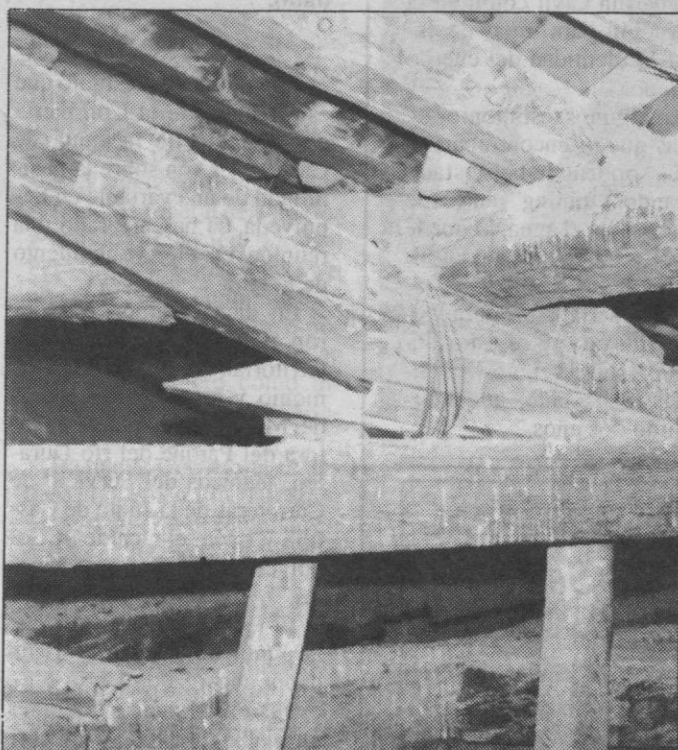
Estado de la cubierta de madera de la iglesia de San Miguel. S.G.
