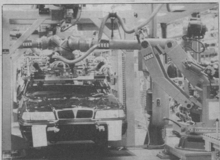
Montaje en la factoría Cowley.
