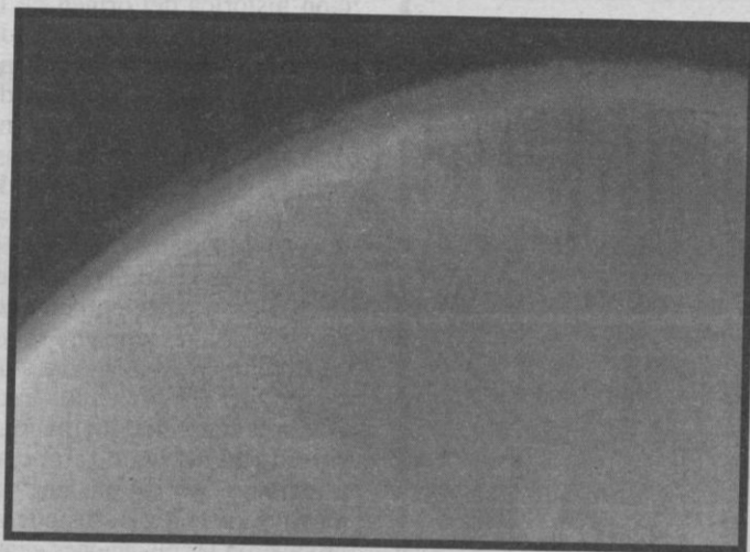
Titán, satélite de Saturno
